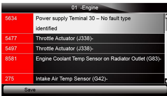
Рис. 4-16 Пример отображения кодов DTC
