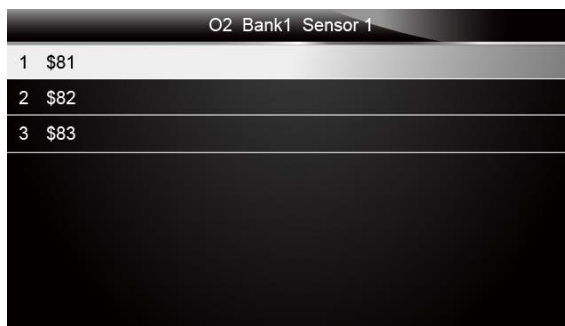
Рис 5-25 Пример экрана теста O2 Банк 1 Датчик 1
